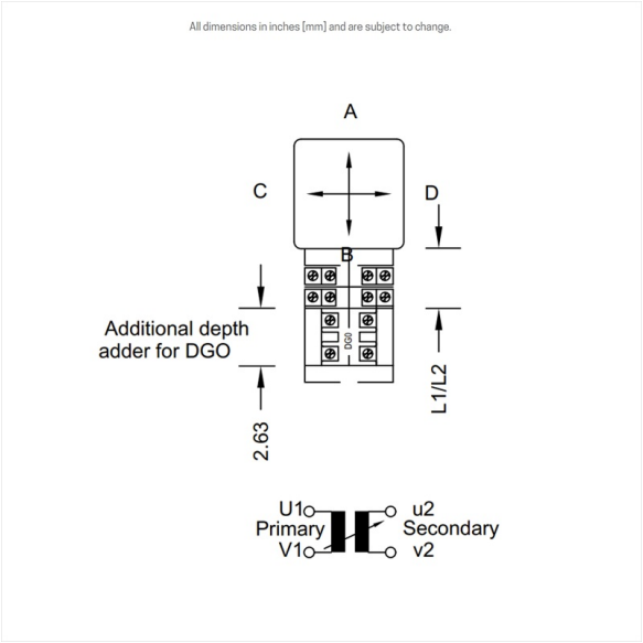
DGO dimensions
