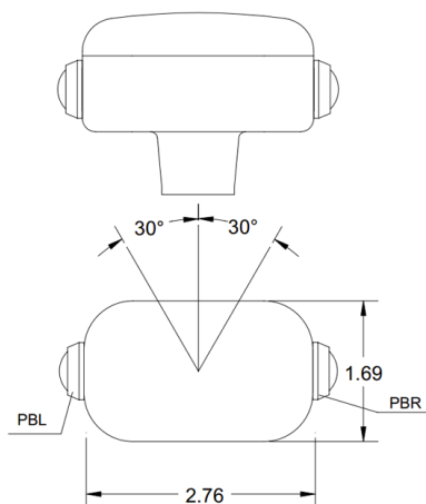
MG13 dimensions
